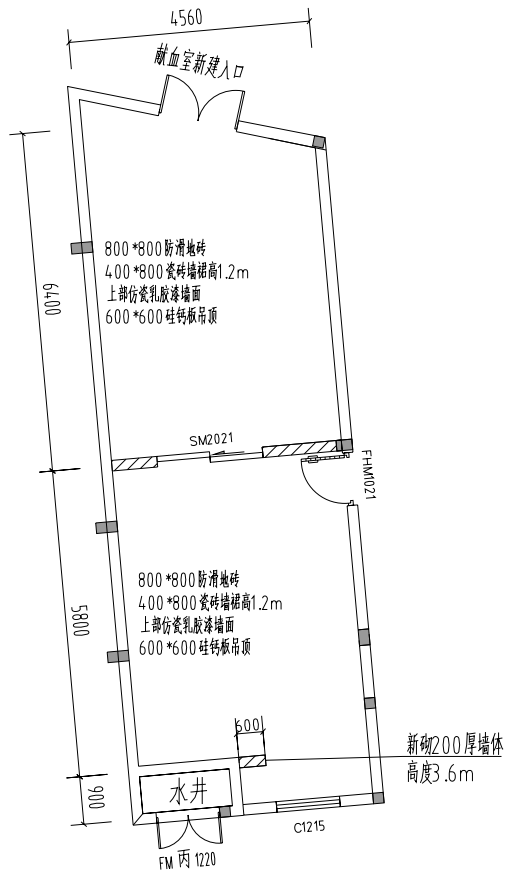
献血室装饰平面图
