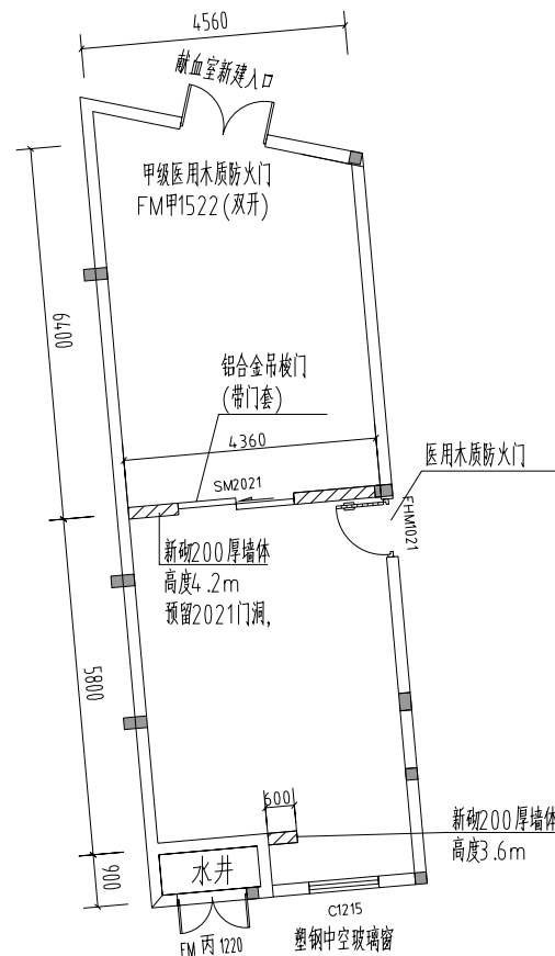
献血室增加墙体平面图
