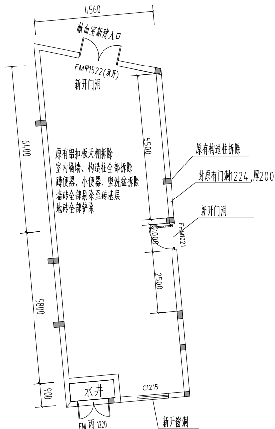
献血室拆除平面图
