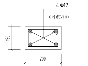
门窗洞口C25过梁大样图
